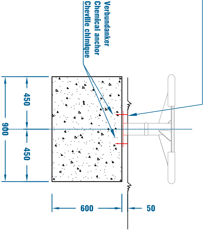
SCHNITT / ELEVATION VIEW / COUPE
