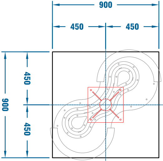
DRAUFSICHT / PLAN VIEW / VUE DE DESSUS
